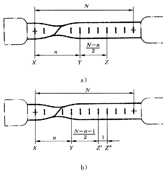
图 F1 移位方法的图示说明
