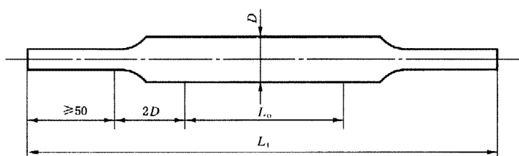
图 D2 管段试样的两夹持头部压扁
