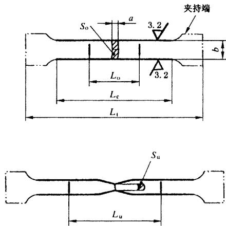
图 13 管的纵向弧形试样(见附录 D)
