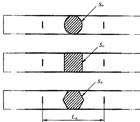
图 11 比例试样(见附录 B)
