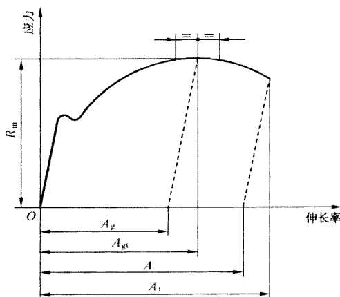
图1 伸长的定义
