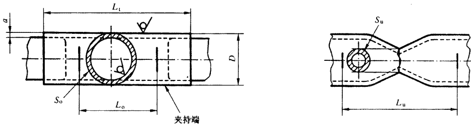
图 14 管段试样(见附录 D)
