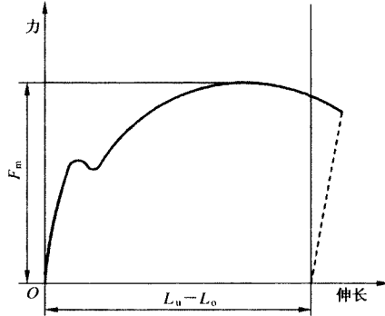
图 8 最大力( F_m )
