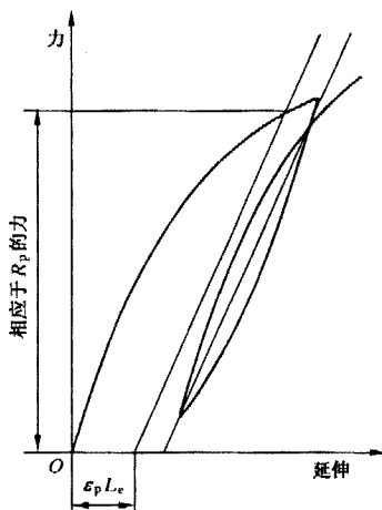
图 7 规定非比例延伸强度( R_p ) (见 15.1)
