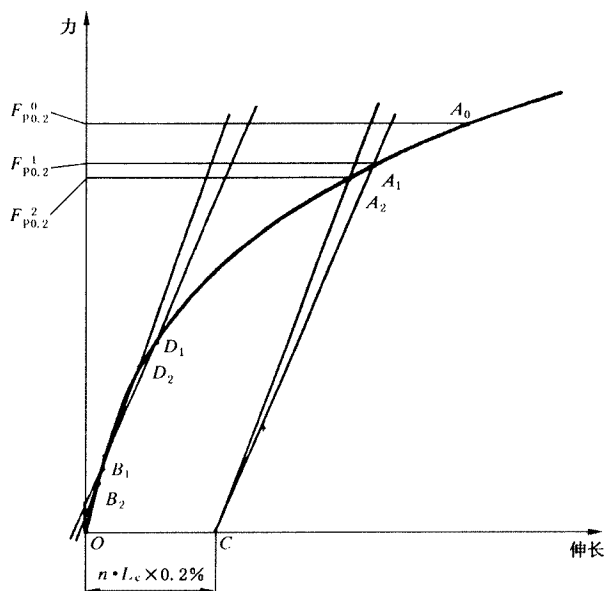
图 H1 逐步逼近方法测定規定非比例延伸强度( R_p )
