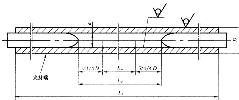
图 D1 管段试样的塞头位置
