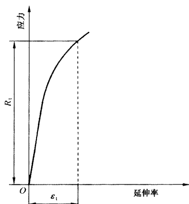
图4 规定总延伸强度( R_t )
